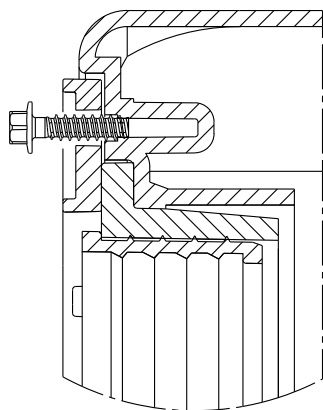
Rys. 18 Śruba w pierścieniu zewnętrznym przed dokręceniem
