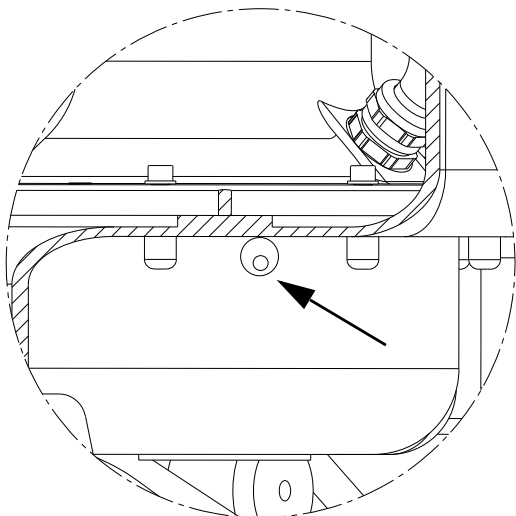
Rys. 31 Otwór odpowietrzający korpus pompy i otwór odpowietrzający w zbiorniku
