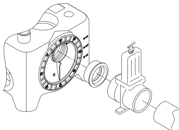
Rys. 21 Montaż zaworu odcinającego
