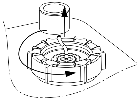
Rys. 33 Demontaż rury kontroli poziomu
