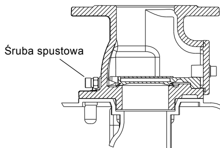
Rys. 4 Zawór zwrotny
