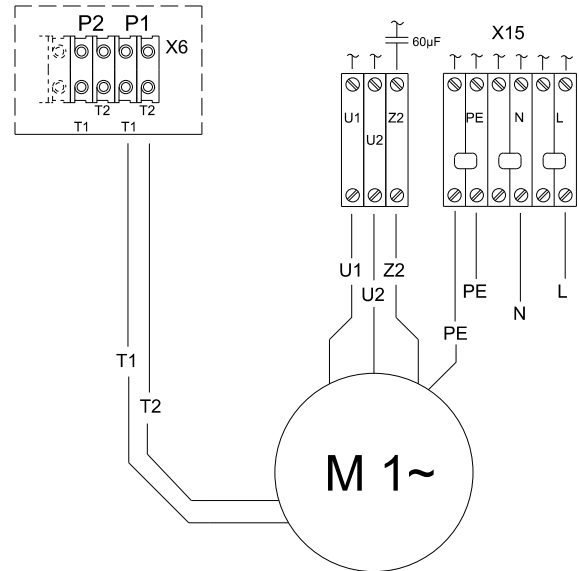
Rys. 25 Schemat połączeń, 1-faz., Multilift M.12.1.4 i M.15.1.4
