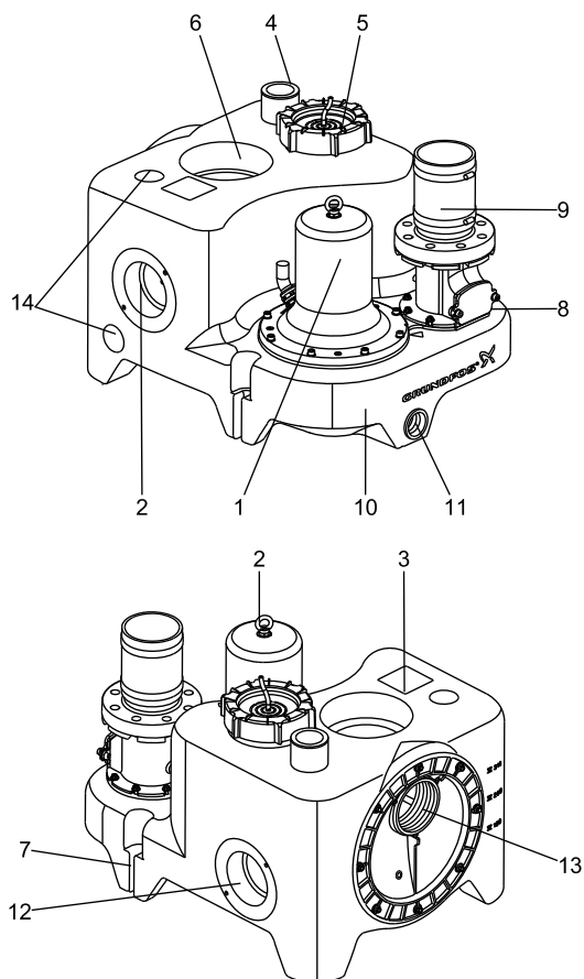
Rys. 1 Multilift M, widok z przodu i z tyłu
