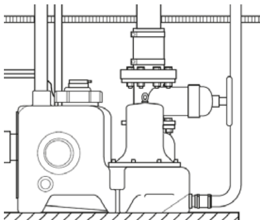
Rys. 22 Zawór odcinający na zaworze zwrotnym
