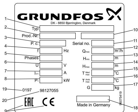
Rys. 2 Tabliczka znamionowa agregatu podnoszącego
