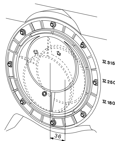
Rys. 17 Opcjonalna obrotowa tarcza z otworem DN 150 umożliwia nastawianie wysokości osi przyłączanej rury w zakresie od 207 do 279 mm nad poziomem posadzki.
