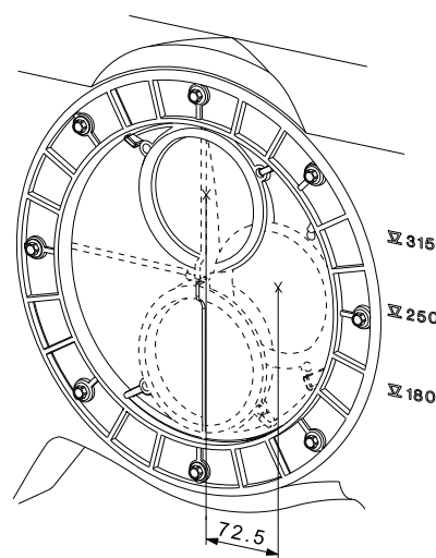
Rys. 16 Obrotowa tarcza z otworem DN 100 umożliwia nastawianie wysokości osi przyłączanej rury w zakresie od 180 do 315 mm nad poziomem posadzki.
