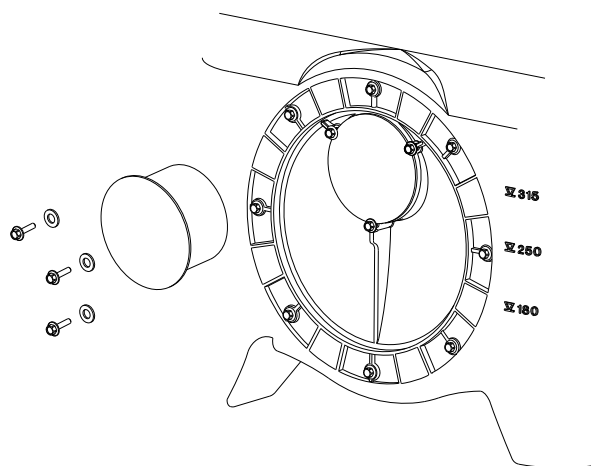
Rys. 19 Zamykanie wlotu tarczy wejściowej
