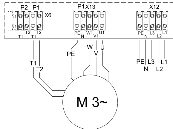
Rys. 26 Schemat połączeń, 3-faz., Multilift M.12.3.4, M.15.3.4
