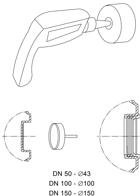
Rys. 20 Wycinanie wzgl. wiercenie otworów przyłączeniowych
