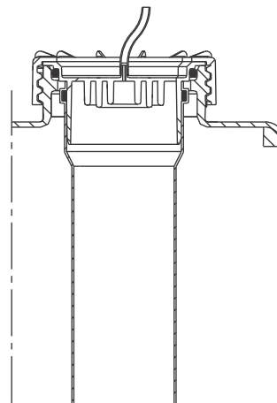
Rys. 5 Nakrętka z wężem i rurą DN 100
