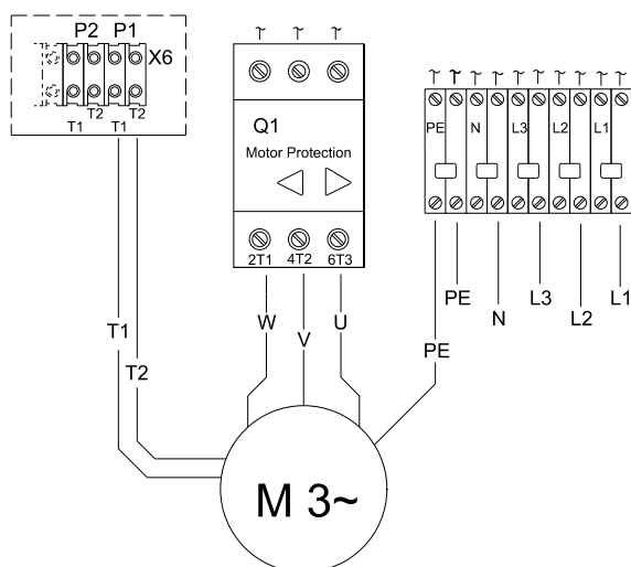
Rys. 28 Schemat połączeń, 3 faz., Multilift M.22.3.4, M.24.3.2, M.32.3.2 i M.38.3.2 z wyłącznikiem ochronnym silnika
