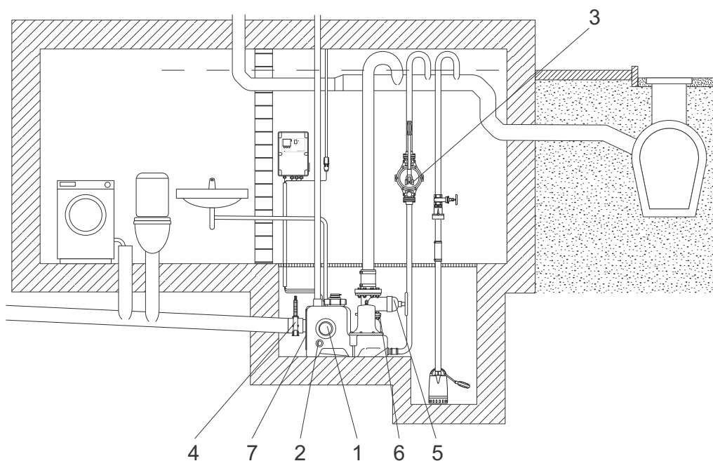
Rys. 15 Instalacja
