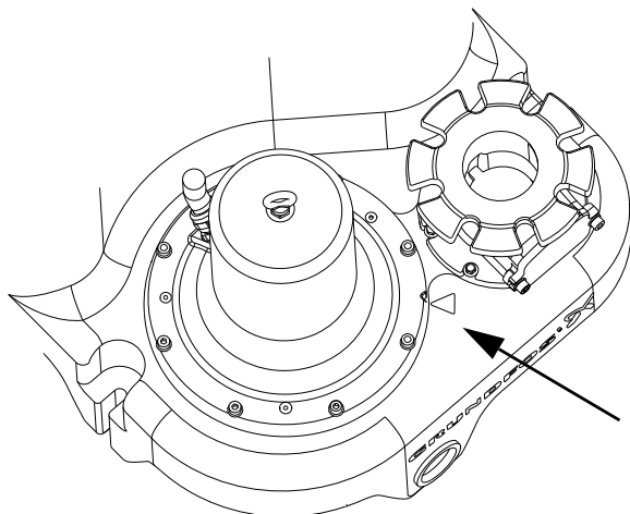
Rys. 32 Znaki ustalające prawidłową pozycję pompy na zbiorniku
