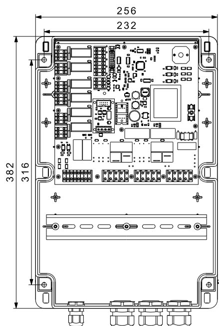
Rys. 24 Montaż sterownika na ścianie
