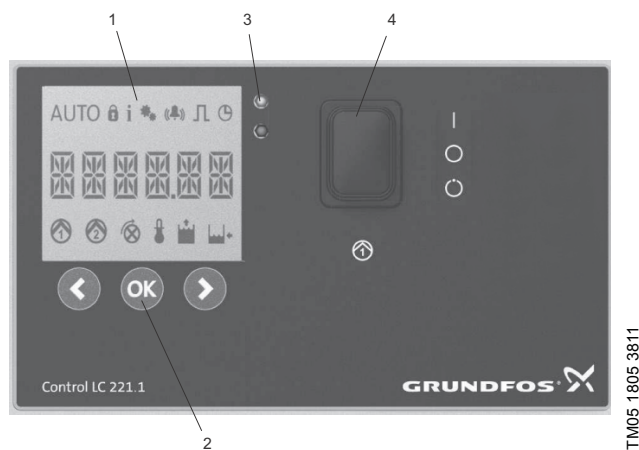
Rys. 9 Panel sterujący
